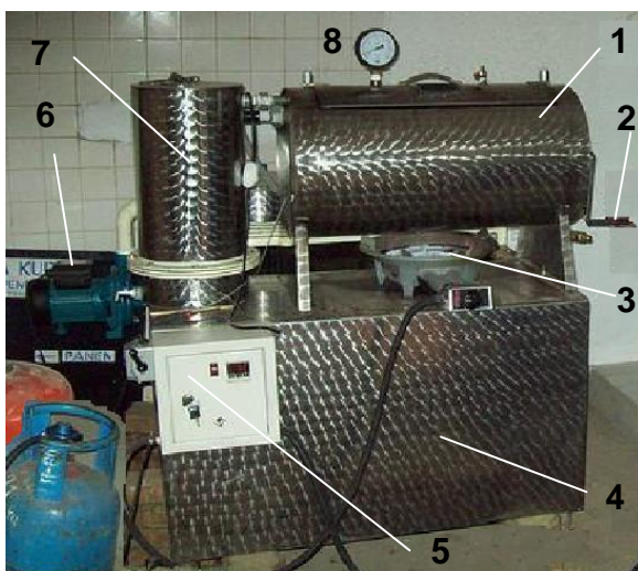
Gambar 1. Mesin Penggoreng Vakum Kapasitas 5 Kg
