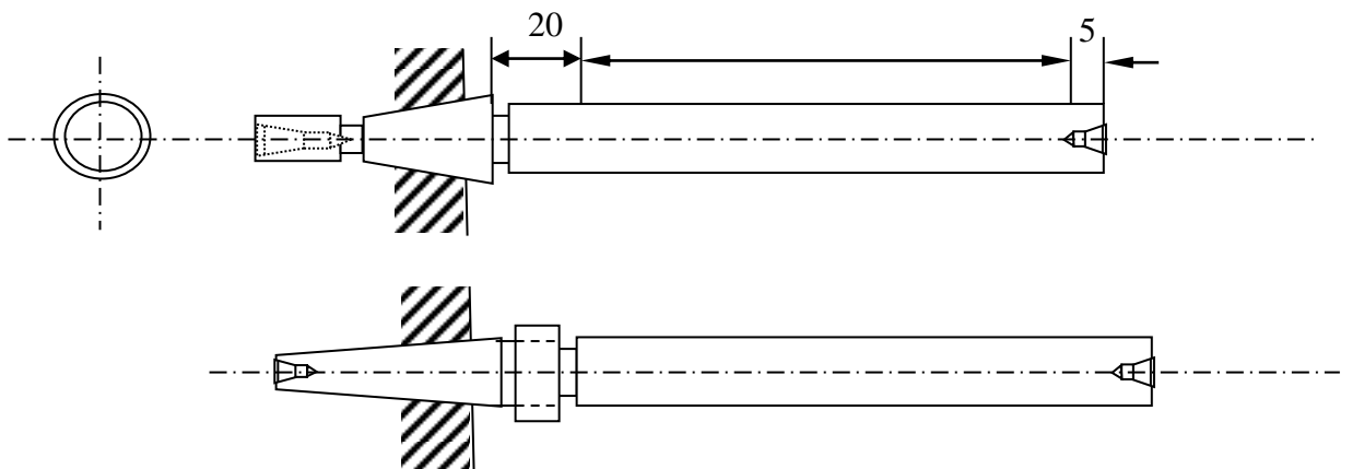
Gambar 2. Mandrel silindrik dan penampung dalamnya
