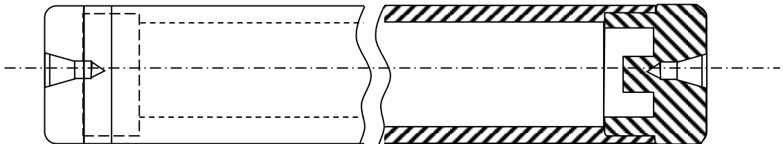
Gambar 2. Mandrel silindrik dan penampung dalamnya
