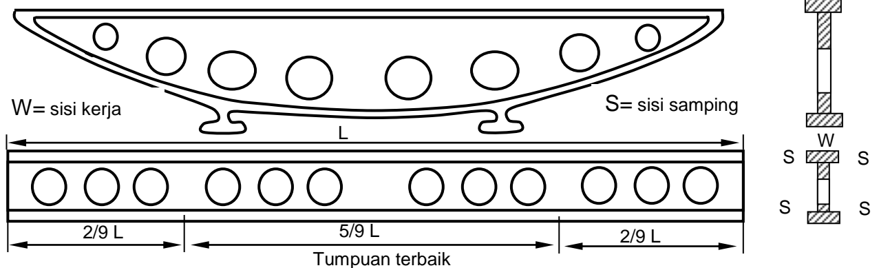
Gambar 4. Pelurus yang dapat dipakai pada pengujian mesin perkakas
