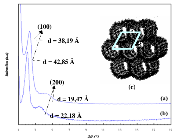
Gambar 1. (a). Difraktogram sinar-x material (a). MCM-41, (b). Ti-MCM-41 dengan [\text{Ti}_8\text{O}_{12}(\text{H}_2\text{O})_{24}]\text{Cl}_8\cdot\text{HCl}\cdot 7\text{H}_2\text{O} sebagai sumber titanium dari dan (c). Parameter kisi MCM-41 ( a = 44,09\text{ \AA} ) & Ti-MCM-41 ( a = 49,48\text{ \AA} ).
