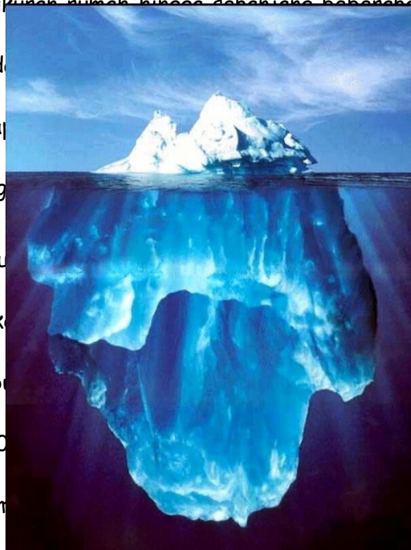
Sebuah gunung es di Newfoundland. Beratnya kira-kira 300.000.000.000 kilogram.
